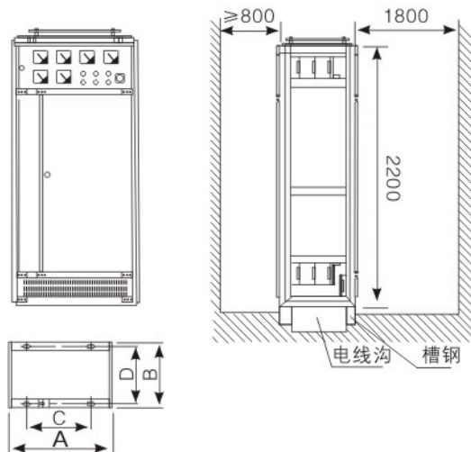
安装示意图
