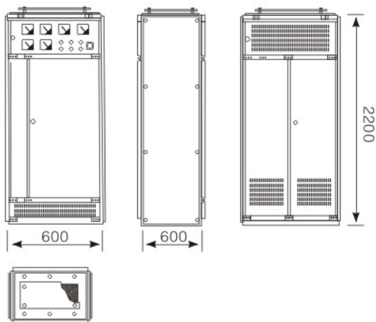
外形示意图
